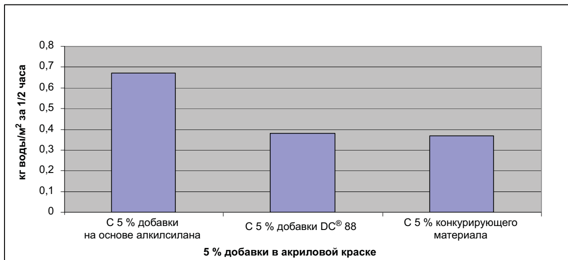
Рис. 1. Добавка Dow Corning® 88 Additive уменьшает поглощение воды пористым субстратом (стандартное испытание DIN 52617)
